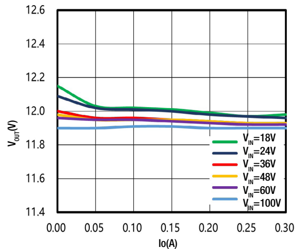
Fig. 23 Vout vs Io
