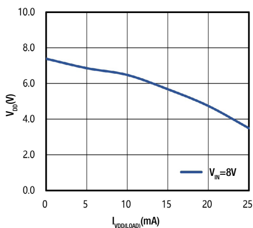
Fig. 9. V DD vs I VDD(LOAD)
