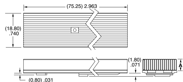
HS-QSFP-D8-1 SHOWN
