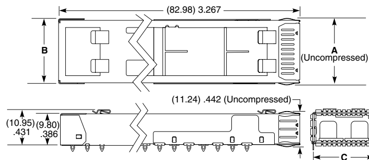
QSFP-D8-1-1-S-F SHOWN
