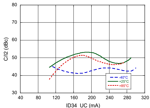
C/I2 vs. LO Bias, RF = 86 GHz
