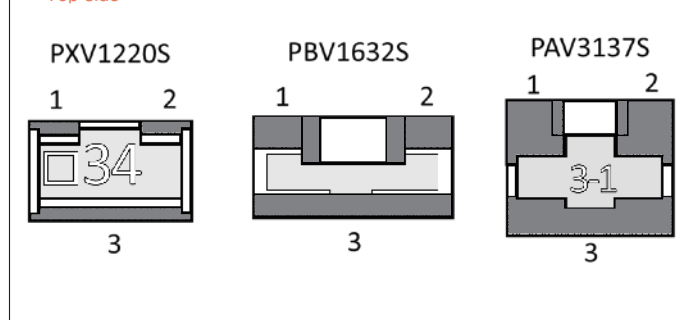
Top side
