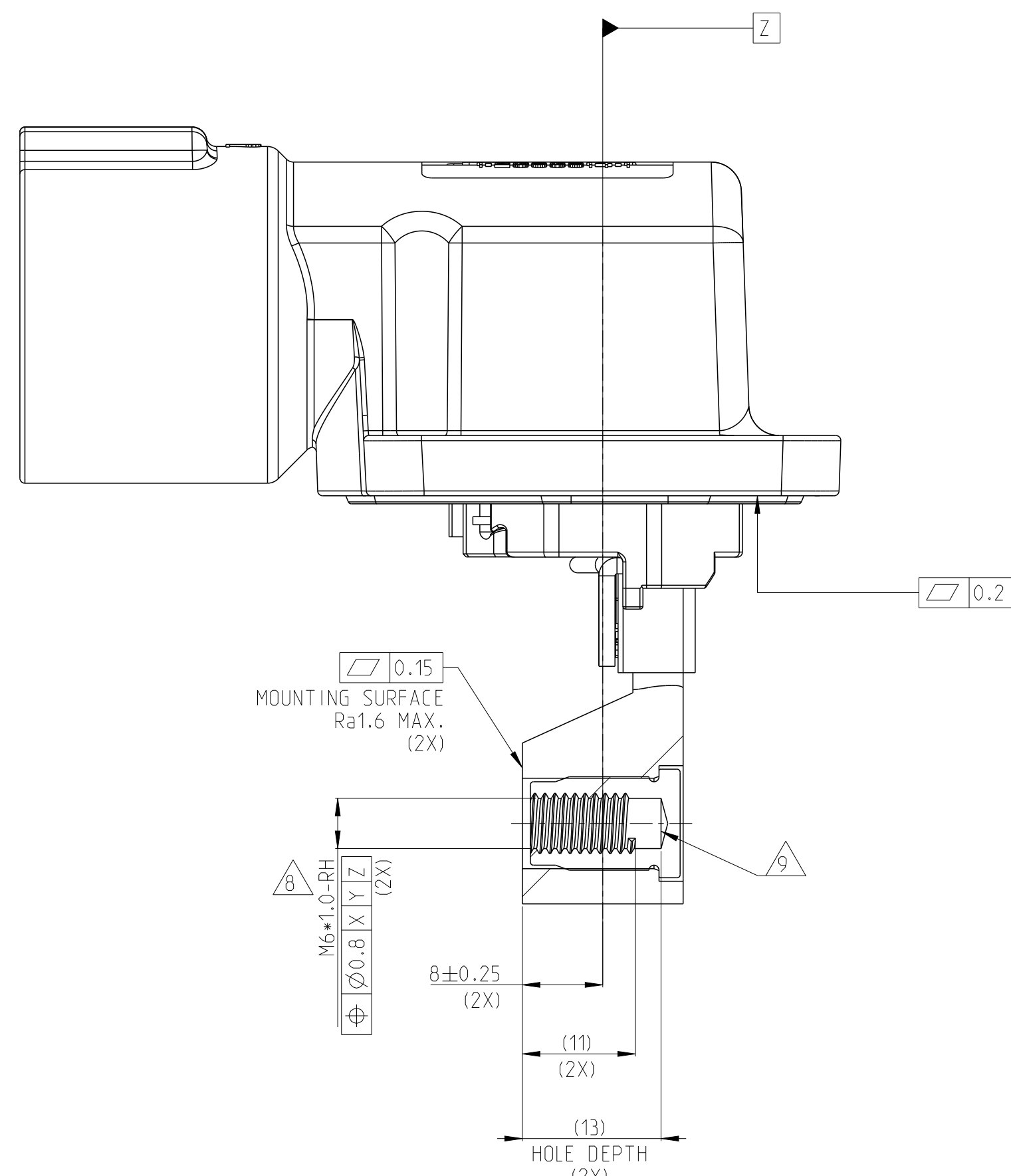
SECTION A-A
