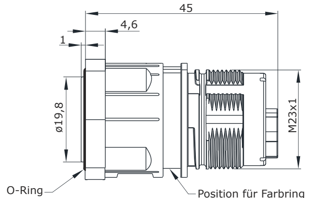
Hauptabmessungen Einbaudose
