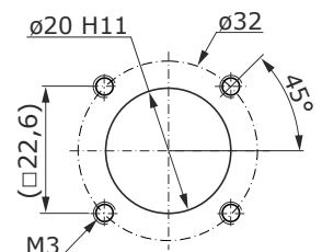
Montagefenster
