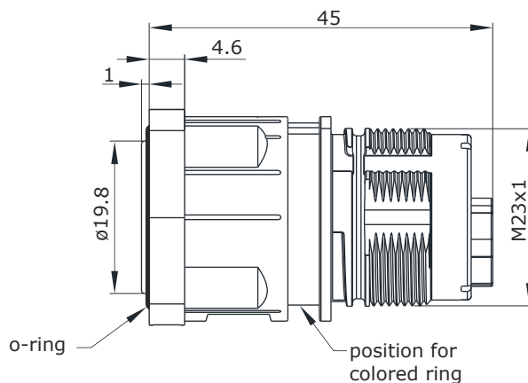
Main Dimensions receptacle
