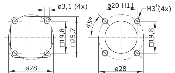
Hauptabmessungen Flansch
