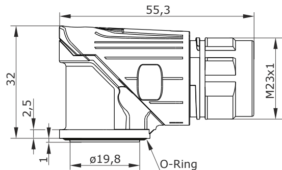
Hauptabmessungen Winkeleinbaudose
