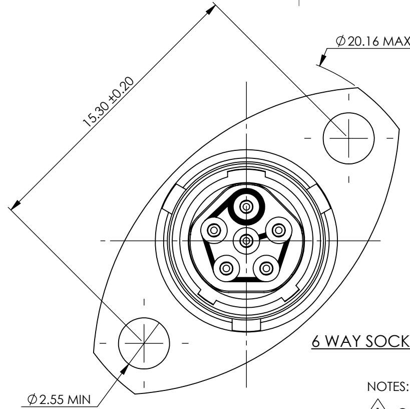
6 WAY PIN INSERT
