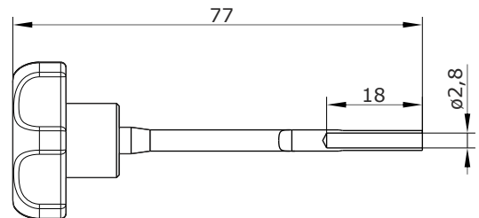
Hauptabmessungen Montagewerkzeug
