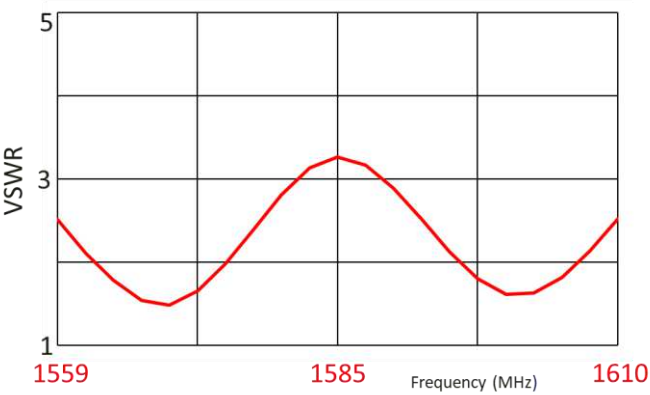
VSWR
