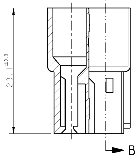
SEZ. PARZIALE A-A PARTIAL SECT. A-A
