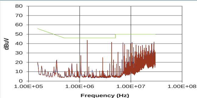
NXJ1S0505(P)T(6)MC (Average)
