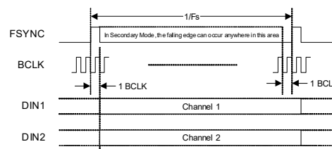
Figure 4-30. TDM Data Format—2 x DIN
