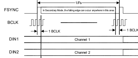
Figure 4-20. TDM Data Format—2 x DIN
