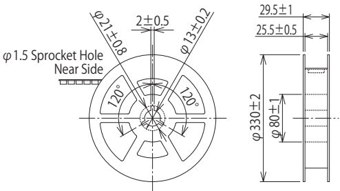
Reel Dimensions
