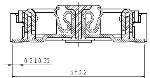
A-A (10:1)
