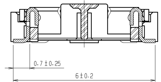
B-B (10:1)
