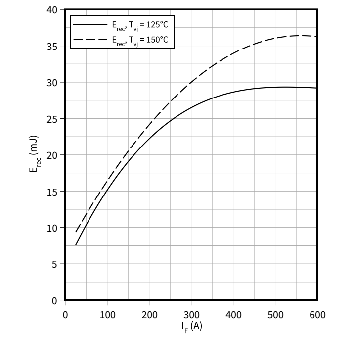
スイッチング損失 (typical), Diode、インバータ E_{rec} = f(I_F) R_{Gon} = 1.3 \Omega , V_{CC} = 600 V
