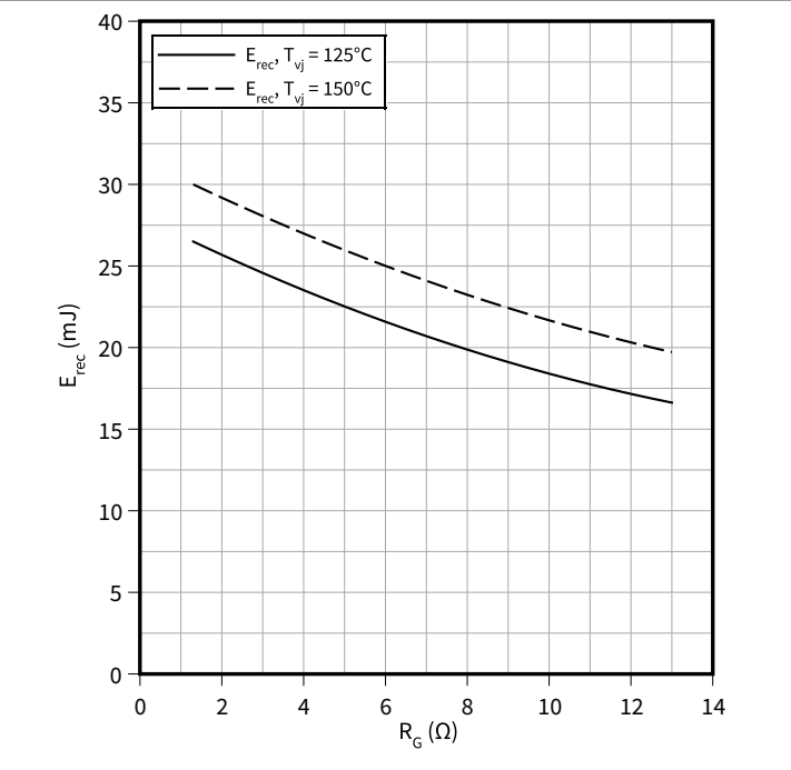
スイッチング損失 (typical), Diode、インバータ E_{rec} = f(R_G) I_F = 300 A , V_{CC} = 600 V
