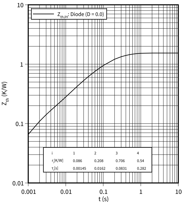
Transienter Wärmewiderstand , Diode, Gleichrichter Z_{th} = f(t)
