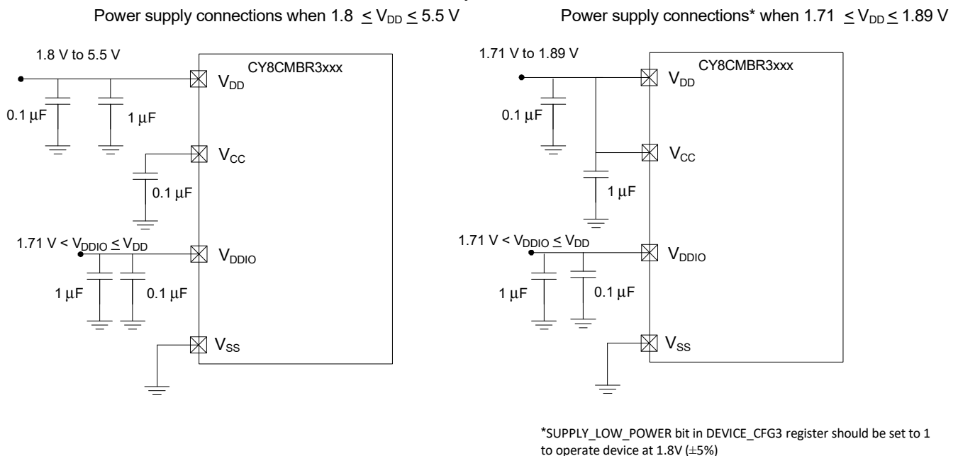
图 15. CY8CMBR3xxx CapSense 控制器的电源连接 [16]
