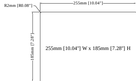
Cutout Dimensions
