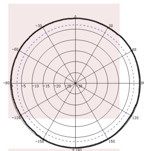
H-Plane: 915MHz
