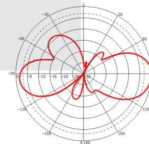
V-Plane: 928MHz
