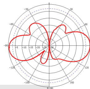
V-Plane: 915MHz
