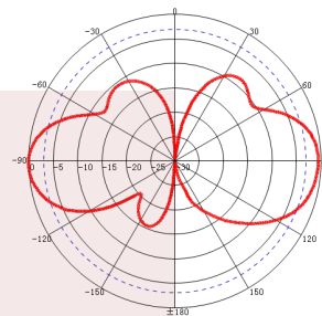
V-Plane: 902MHz
