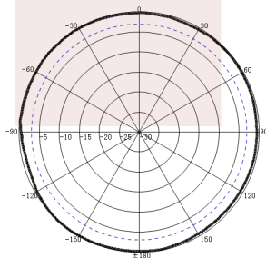
H-Plane: 928MHz
