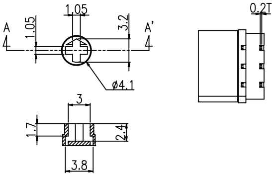
Section A-A' ACTUATOR
