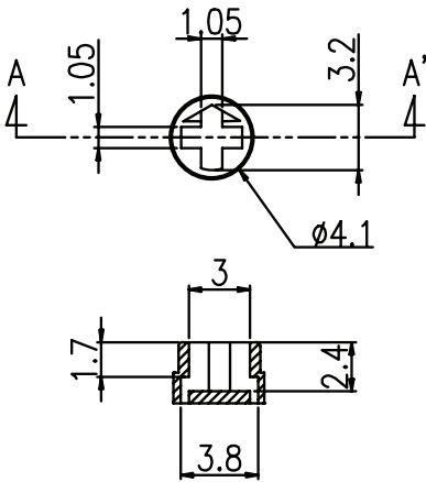
Section A-A' ACTUATOR
