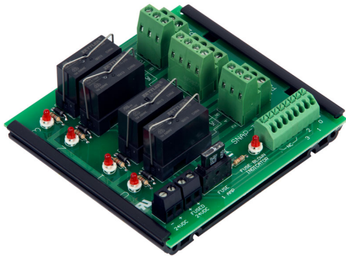
SNAP-TEX-MR10-4
