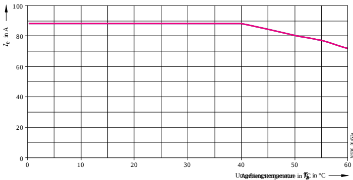
— I IEC Strom nach IEC 947-4-3 bei Einzelaufstellung und Dicht-an-Dicht-Montage
