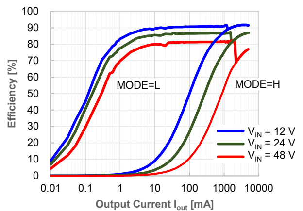
fosc = 600 kHz
