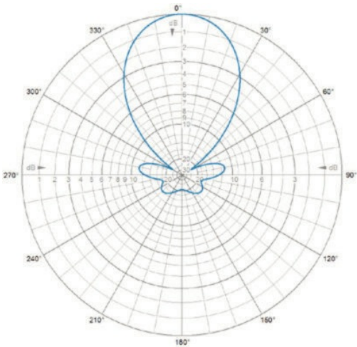
H-Plane | 445 MHz
