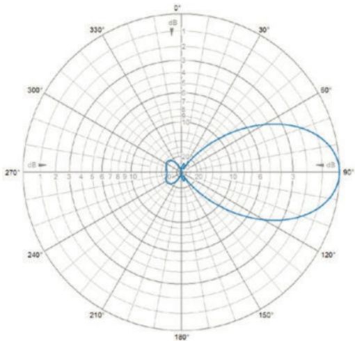
E-Plane | 445 MHz
