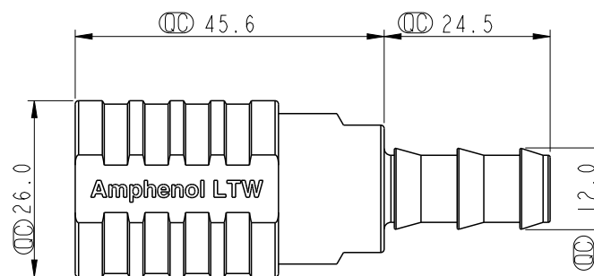
Socket
