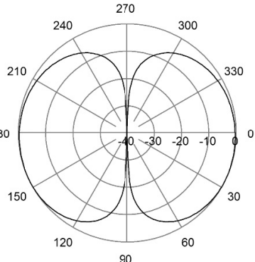
E-Plane | 300 MHz
