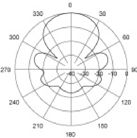
H-Plane | 340 MHz
