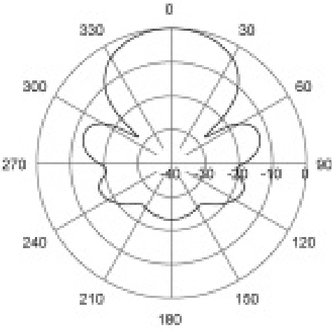
H-Plane | 330 MHz
