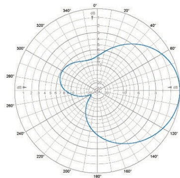
E-Plane | 425 MHz
