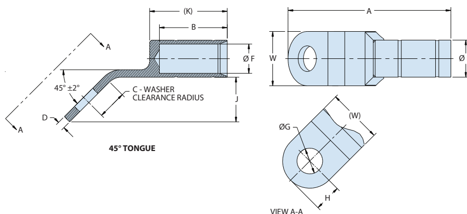
VIEW A-A
