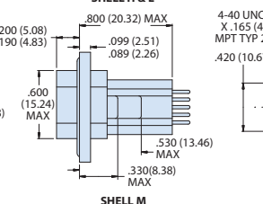
791-069 Dimensions
