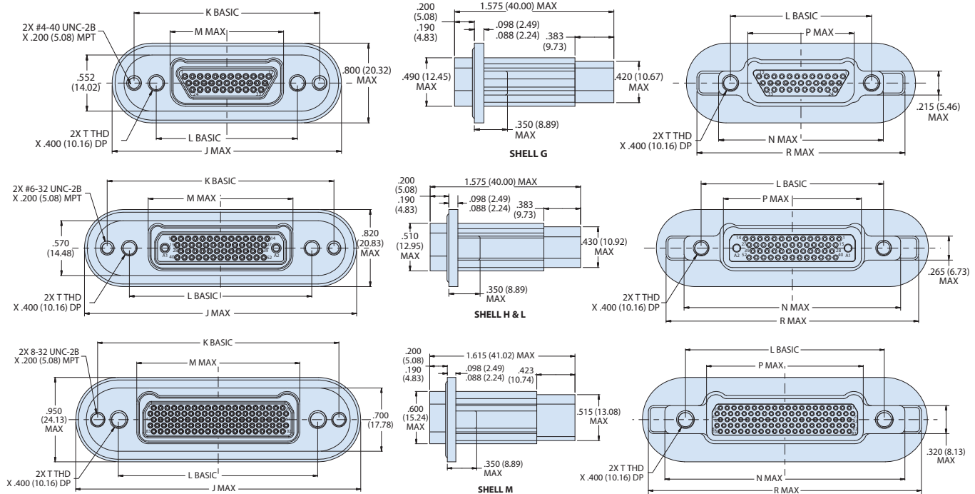
791-070 Dimensions
