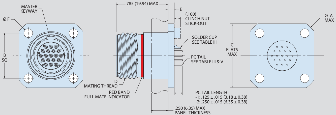
Dimensions
