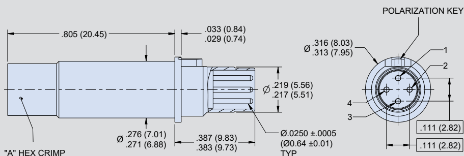
Pin Contact 854-047
