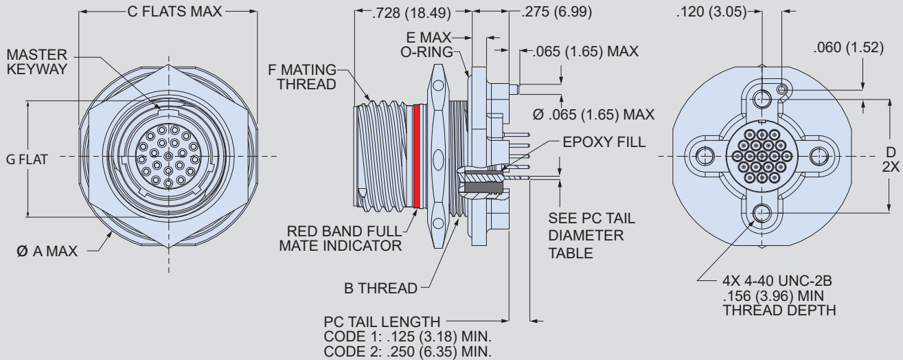
806-021 Receptacle Dimensions
