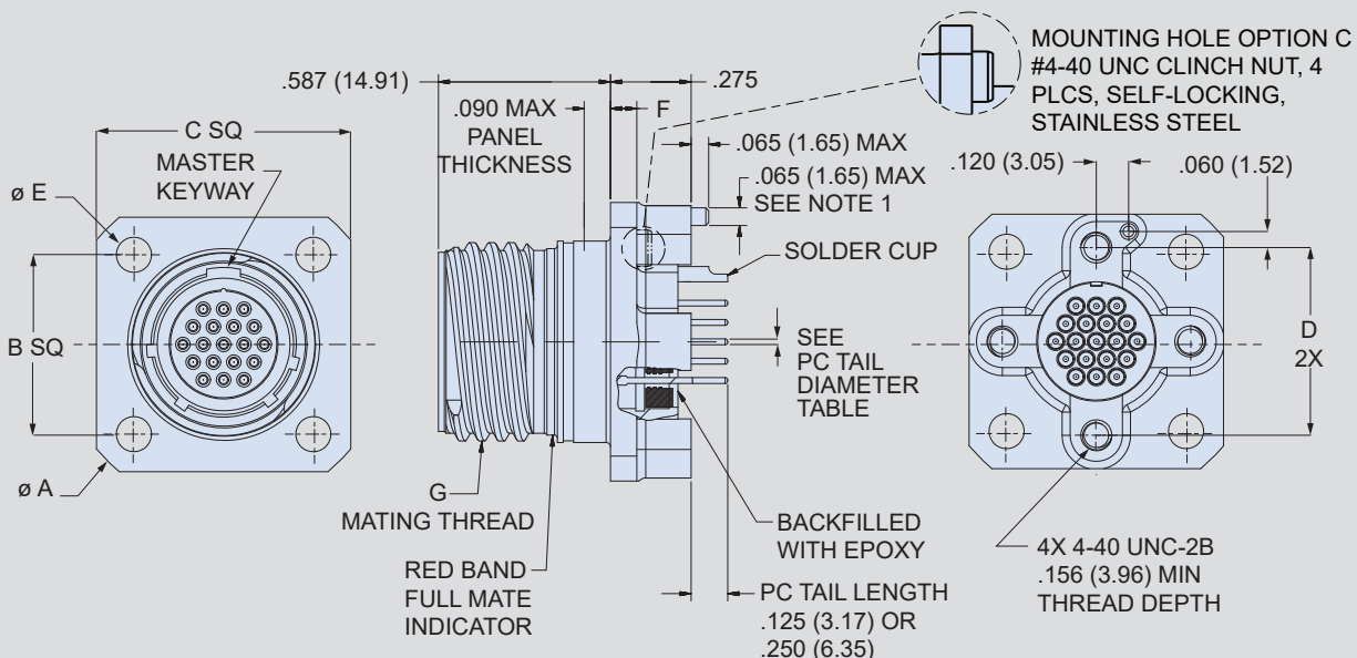
806-022 Receptacle Dimensions
