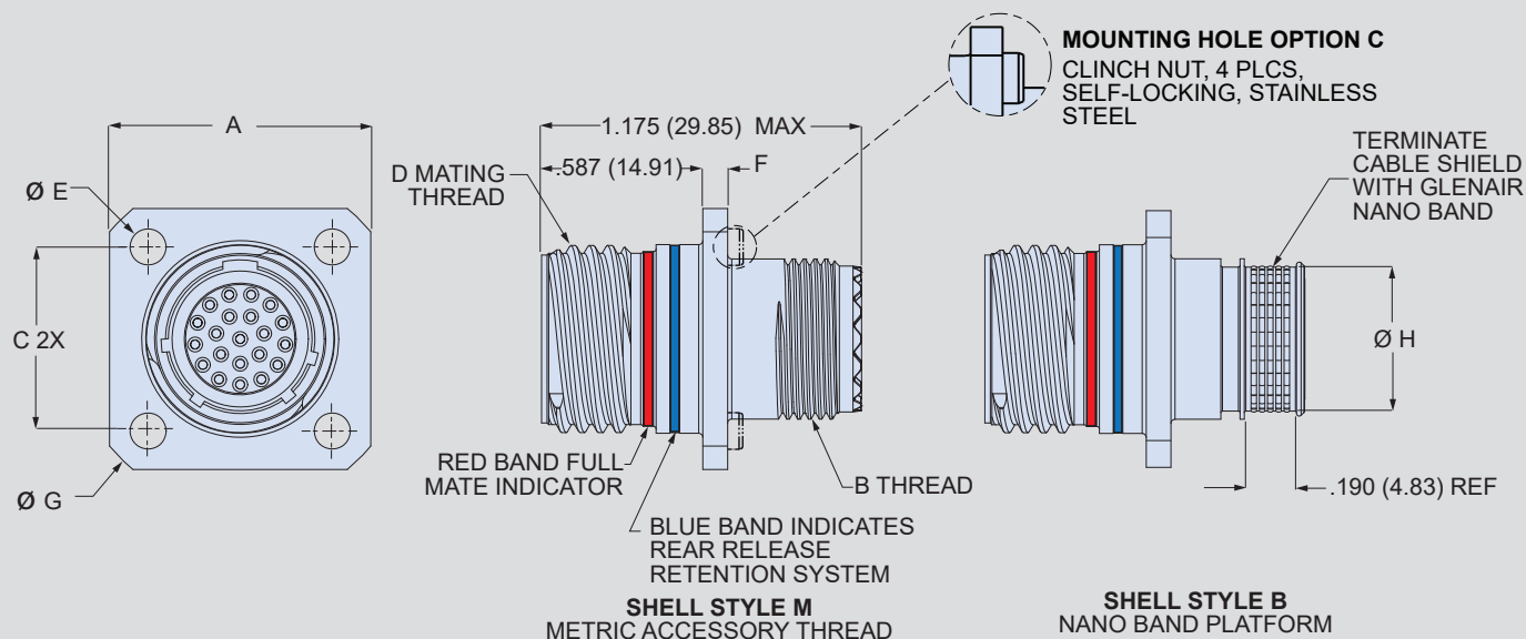
806-013 Receptacle Dimensions
