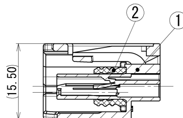
SEC. A-A
