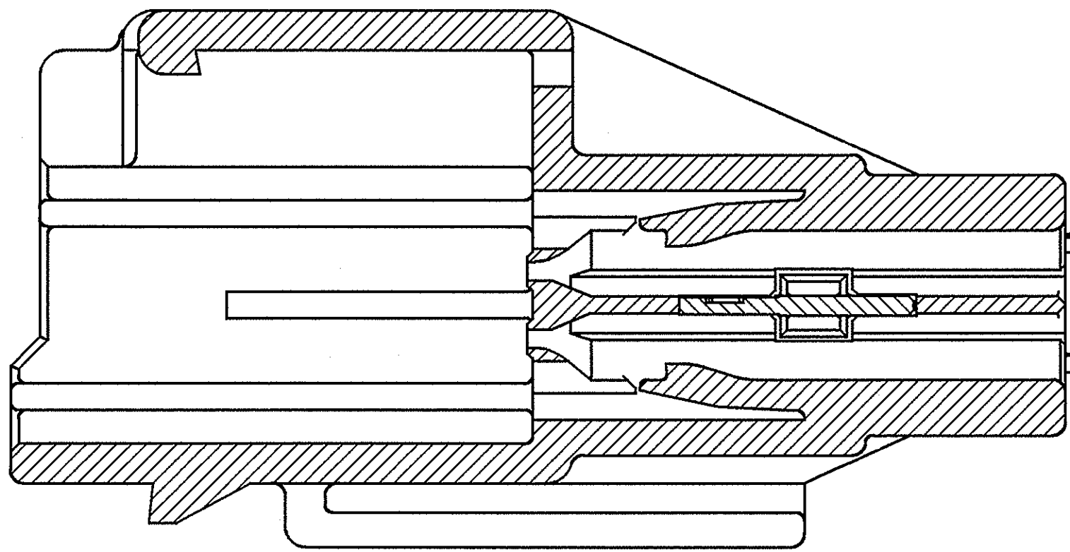
SECTION A-A
