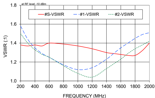
VSWR
