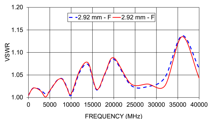
KFFL-KF50+ VSWR
