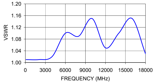
BW-S20W5+ VSWR
