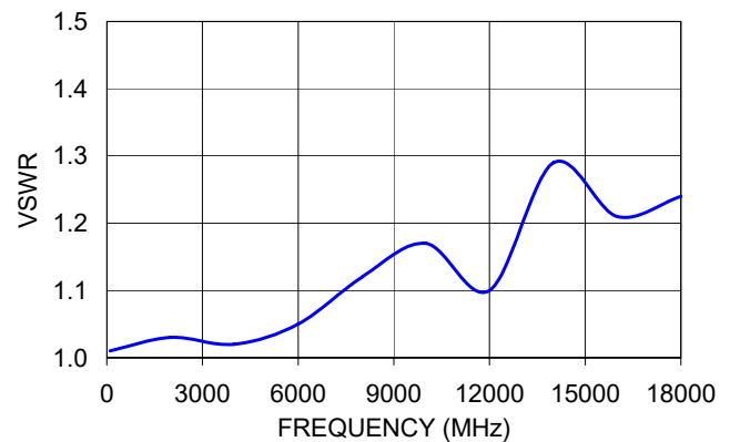
BW-N4W5+ VSWR
