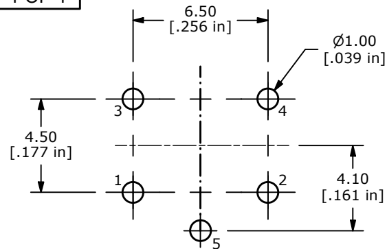
P.C. LAYOUT
