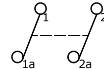
▲ CIRCUIT: DPST ON-OFF
