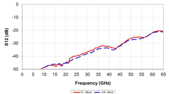
S12
