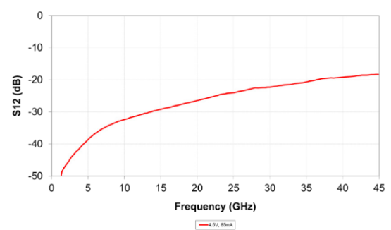
S12
