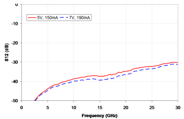
S12
