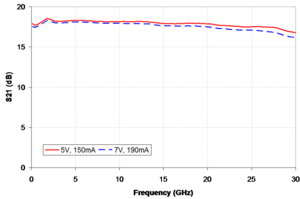
S21
