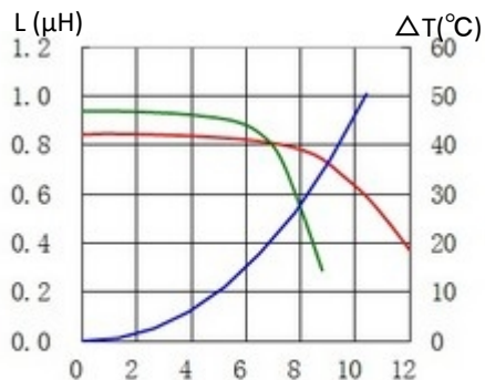
1. CDRH70D45BT150NP-R80NC
