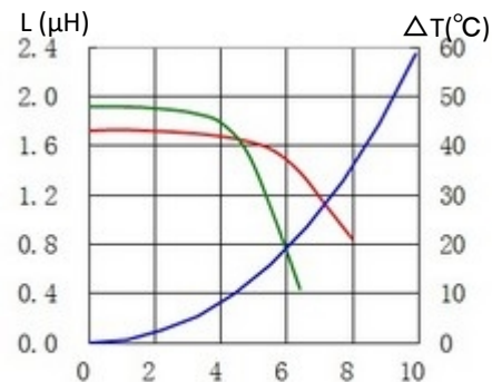
3. CDRH70D45BT150NP-1R5NC
