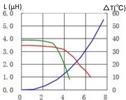
5. CDRH70D45BT150NP-3R3NC
