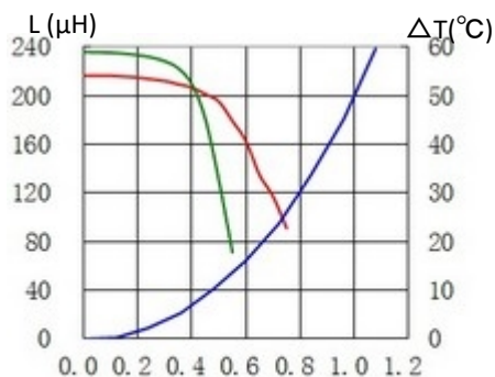
16. CDRH70D45BT150NP-221MC
