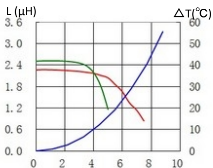
4. CDRH70D45BT150NP-2R2NC
