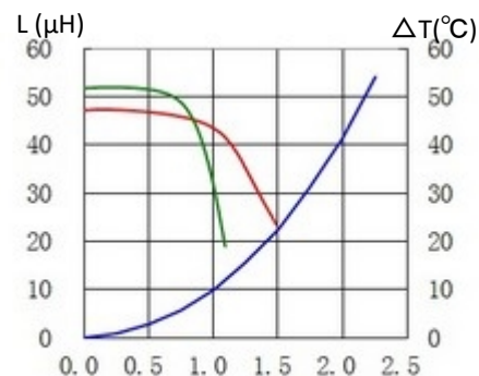
12. CDRH70D45BT150NP-470MC
