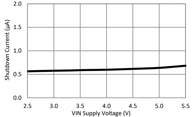
Shutdown Supply Current vs. VIN Voltage (EN = Low)
