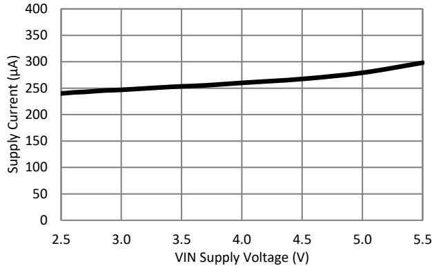
No-Load Supply Current vs. VIN Voltage (EN = High)
