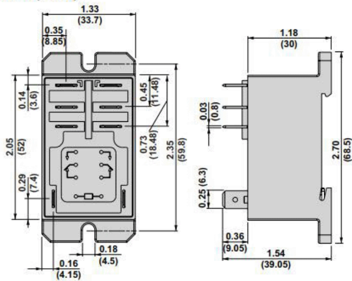
DPDT (2 CO):
