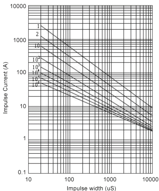
10 mm 820K - 751K
