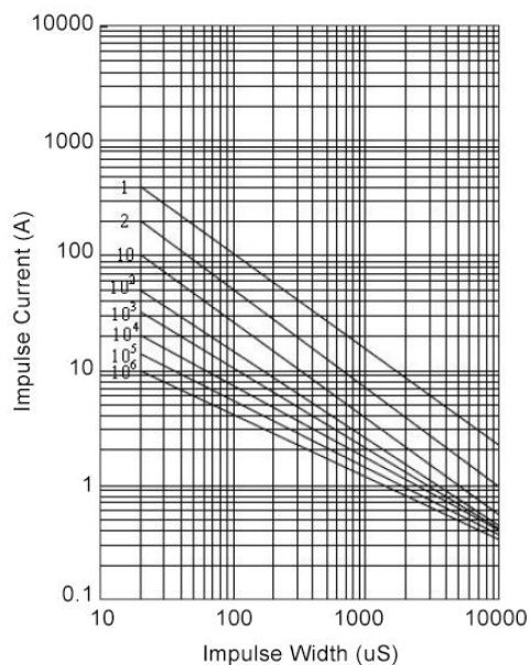
7 mm 820K - 471K
