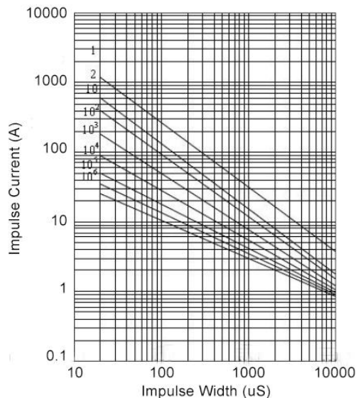
7 mm 820K - 471K
