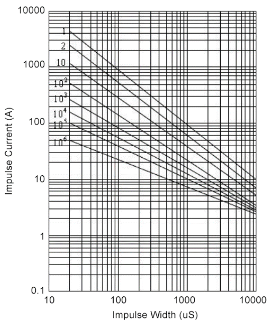
14 mm 821K - 182K
