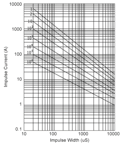
20 mm 821K - 182K
